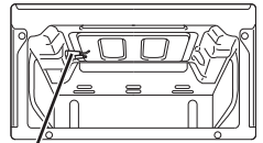
電極（點火針）
