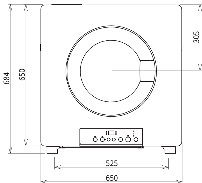
正面圖
